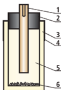
Figura 1. Ejemplo de aplicación de un electrodo de medición no polarizable (electrodo de cobre/sulfato de cobre) para adquirir un potencial dentro del electrolito (vista de sección transversal)
