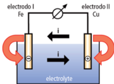
Figura 2. Celda galvánica: hierro/cobre
