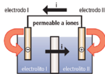
Figura 3. Celda de concentración
