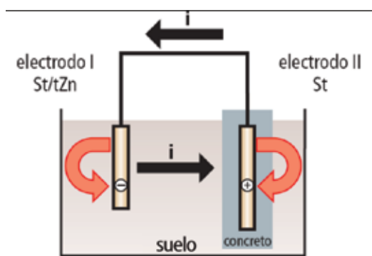
Figura 5. Celda de concentración: acero galvanizado en suelo/acero (negro) en hormigón
