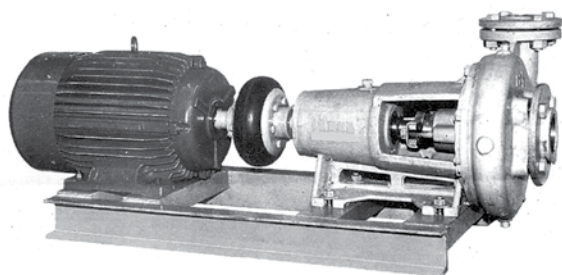
Figura 2. Bomba acoplada con un acoplamiento elástico
