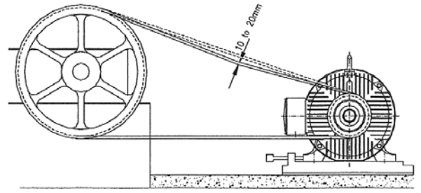
Figura 9. Tensión de la correa
