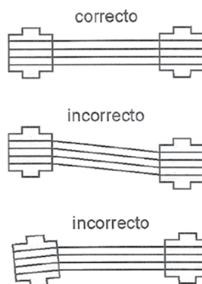
Figura 12. Alineación de acoplamiento
