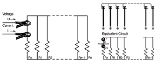
Figura 10: conexiones para la medida sin picas de la impedancia del electrodo
