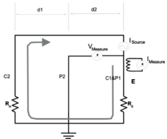
Figura 5. Circuito eléctrico de la medida.
