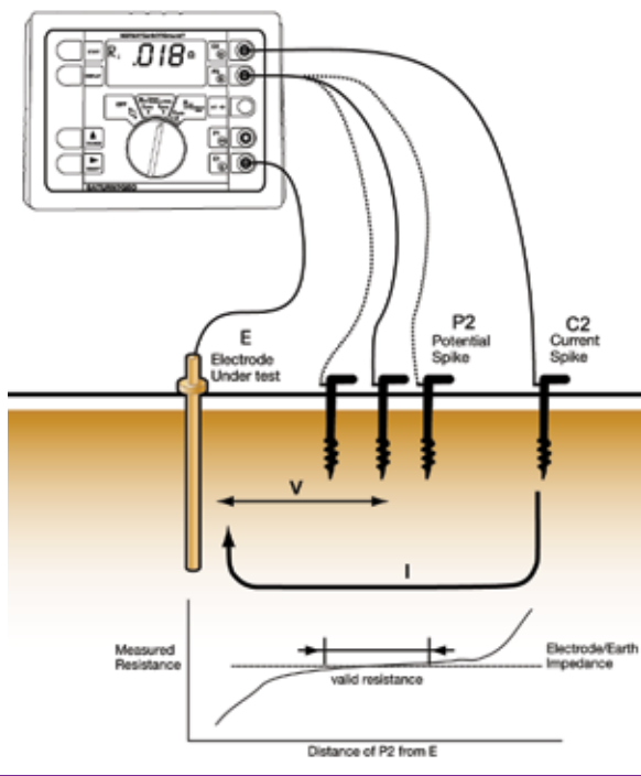
Figura 4. Esquema de conexión del telurómetro.
