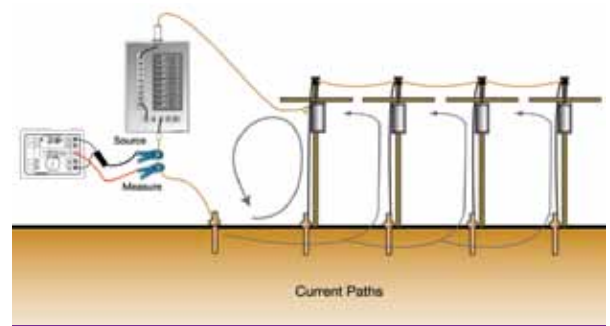
Figura 11. Rutas de corriente de comprobación en el método sin picas
