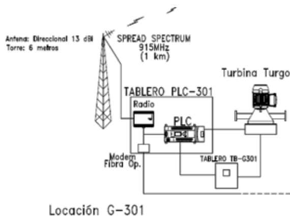
Figura 2. Diagrama de sistema de la turbina Turgo.
