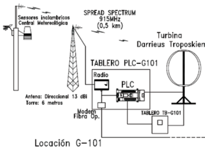
Figura 3. Esquema para la turbina Darrieus.
