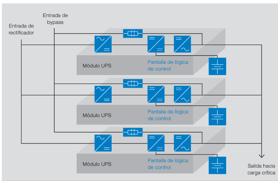
Figura 1. Cada módulo UPS tiene el hardware y el software necesarios para un funcionamiento autónomo; no se comparten elementos críticos.
